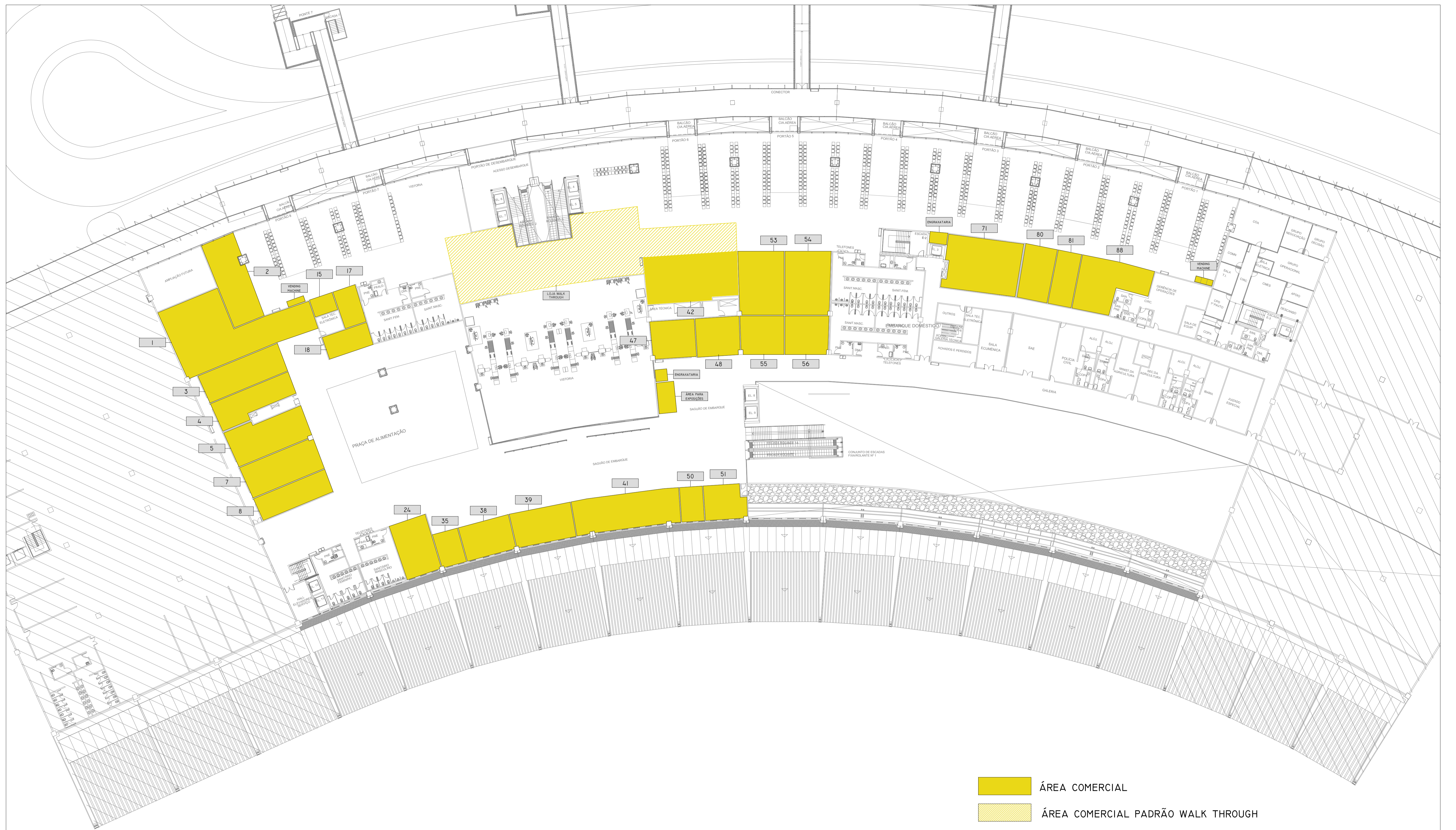
PLANTA BAIXA - 1º PAVIMENTO ESCALA 1:350
